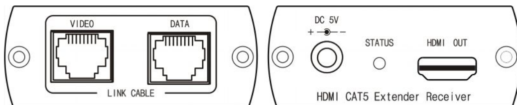
Рис.4 Панель подключения HE01ER
