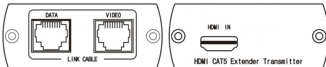
Рис.3 Панель подключения HE01ET
