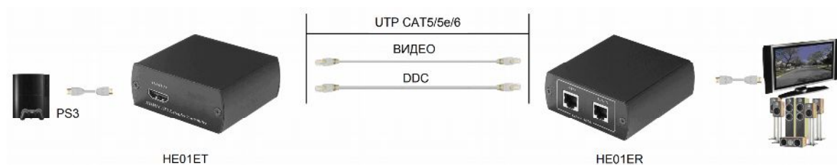
Рис.2 Структурная схема подключения
